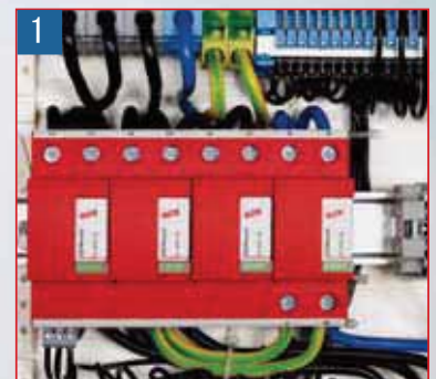
安装在配电柜中的DEHNventil® modular DEHNventil® modular in a power supply cabinet
